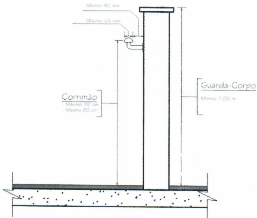
Figura 1- Altura do guarda corpo em patamares internos (fonte RTCBMRS nº 11- Parte 1)
