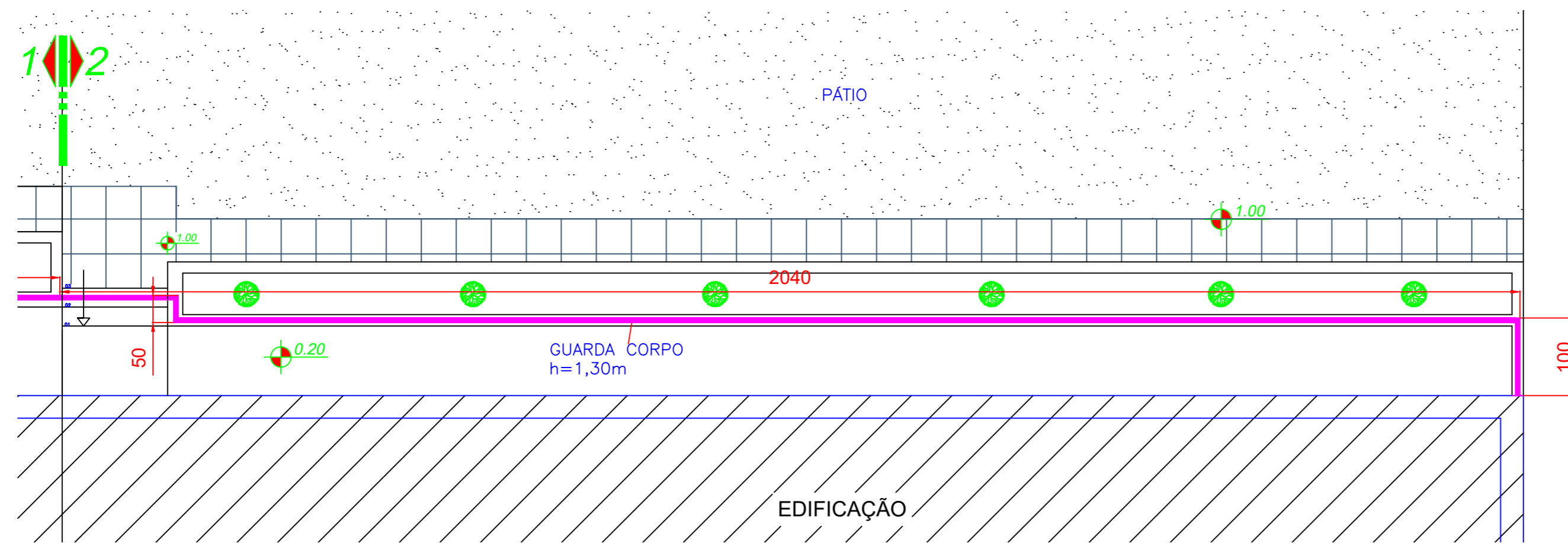
PLANTA BAIXA - PARTE 2
