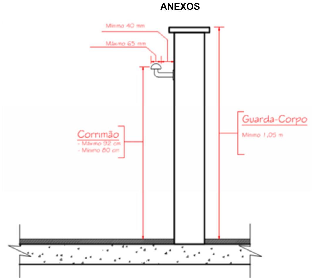
Figura 1- Altura do guarda corpo em patamares internos (fonte RTCBMRS nº 11- Parte 1)
