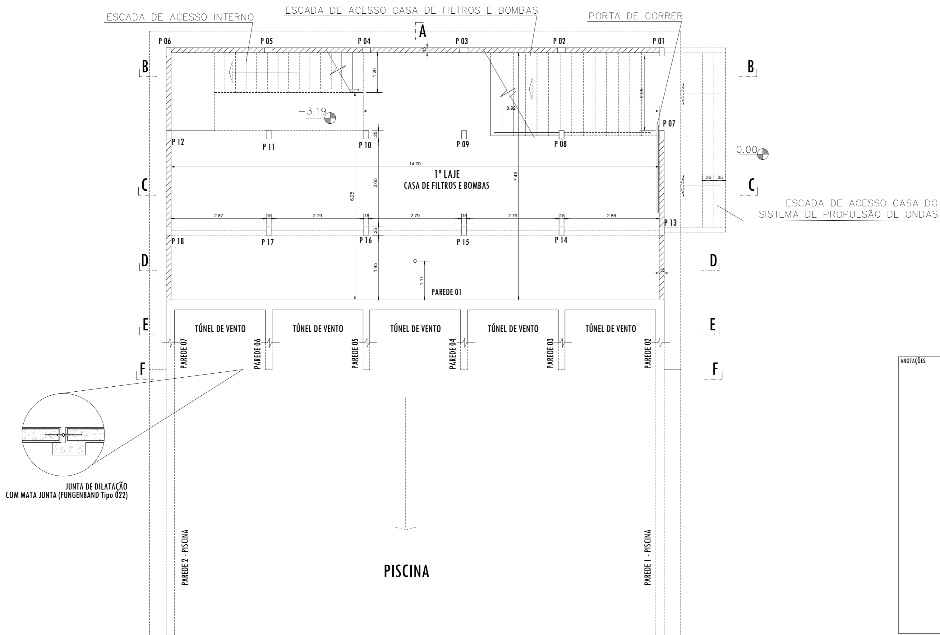
PLANTA "2" PISCINA COM ONDAS
